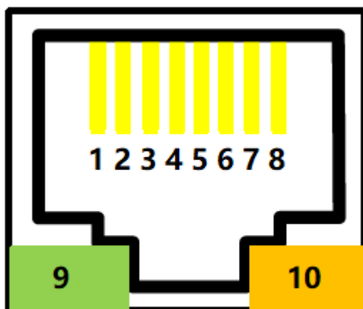
Figure 3. Elfin-EE10 RJ45 接口引脚定义
